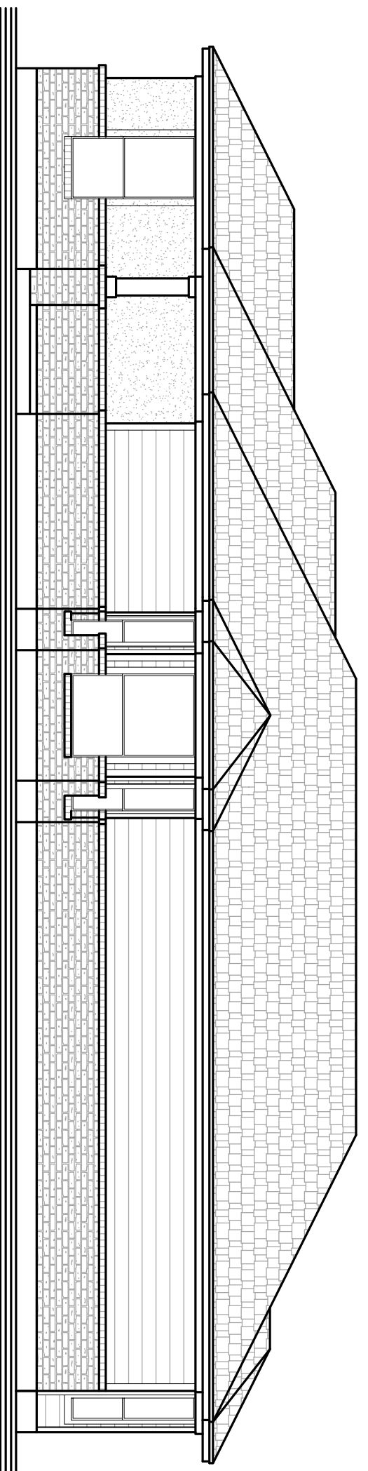
RIGHT ELEVATION
