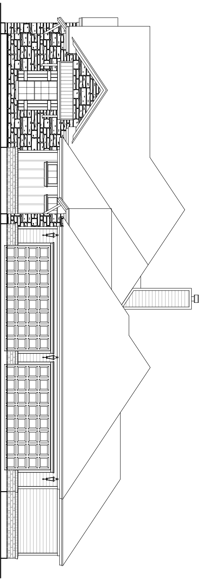
RIGHT ELEVATION
