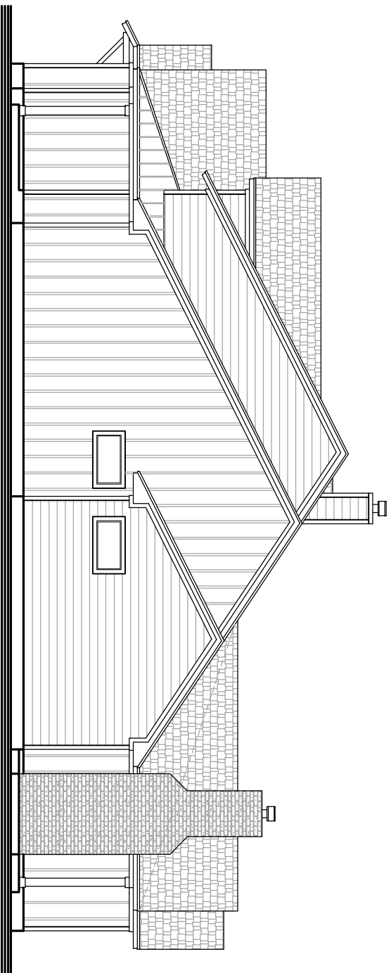
RIGHT ELEVATION
